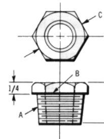
AD-124-.8, AD-125-.8, AD-584-.8, AD-585-.8
